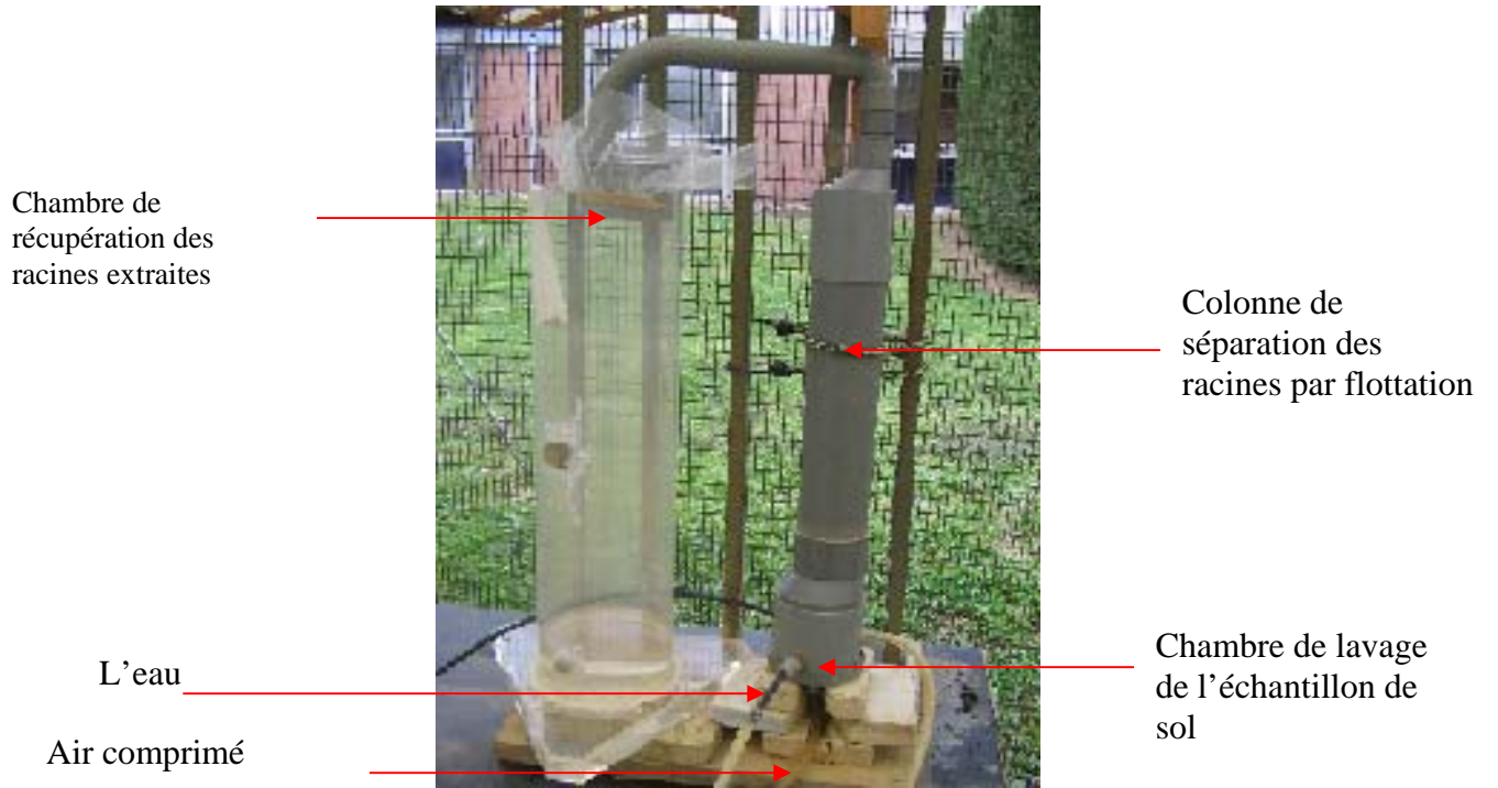
Figure 6. L'appareil de séparation des racines
