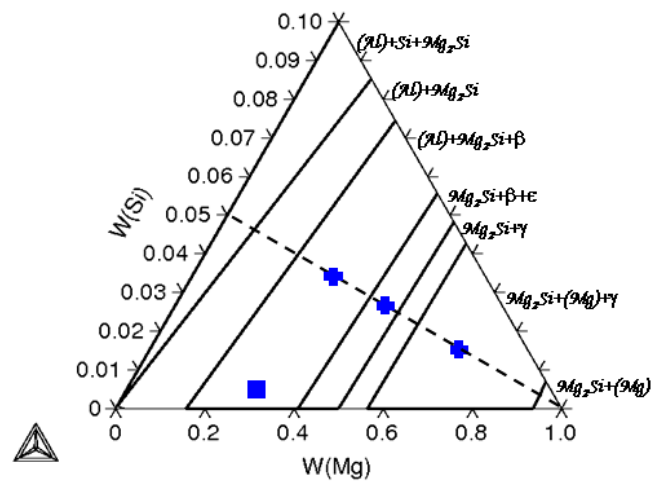
Figure I-1 : Section isotherme à 300 °C du système Al-Mg-Si.
