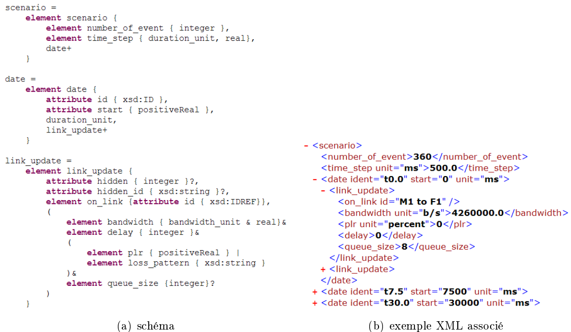
FIG. 4.16: Extrait d'un scénario d'émulation pour la partie scénario
