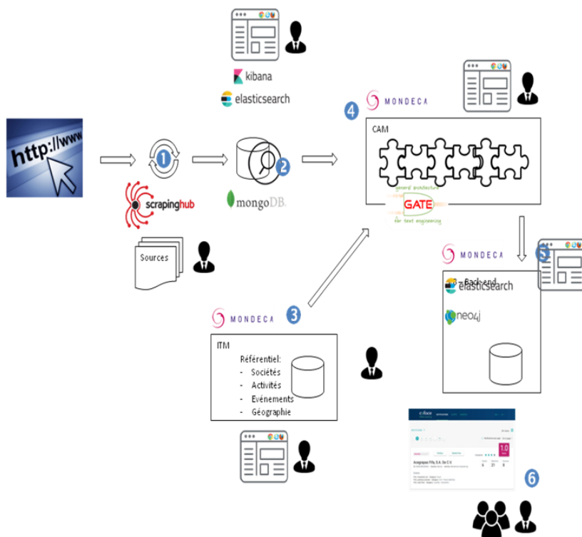
Figure 4.1 – Architecture de la solution d'identification de risques, combinant des systèmes de règles et FastText. Le système suggère des alertes avec un score à valider par un expert métier.
