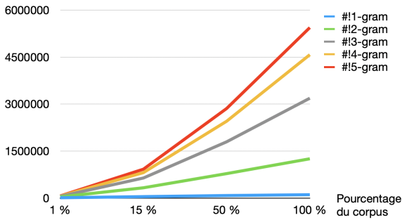
FIGURE 4 – Nombre de n-grammes uniques en fonction du pourcentage du corpus considéré et pour différents gram-mes.
