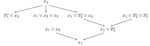
FIGURE 2 – Explication de la clause (x_1) dans \phi
