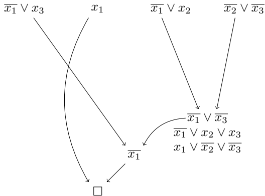
FIGURE 5 – Adaptation de la deuxième réfutation
