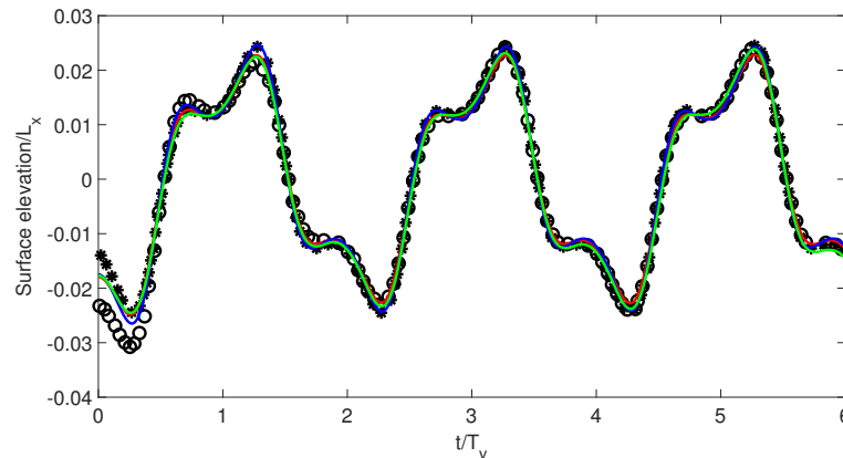
(a) k = 48 \text{ mm}^{-1} (subharmonic case)
