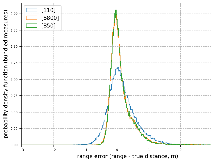
Figure 4.4 – Distribution des erreurs de ranging en fonction du débit utilisé.
