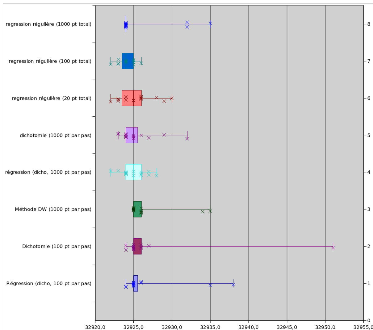
Figure 4.2 – Dispersion des résultats pour le calcul du délai d'antenne
