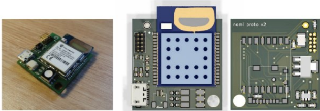
Fig. 5. Nomi nodes
