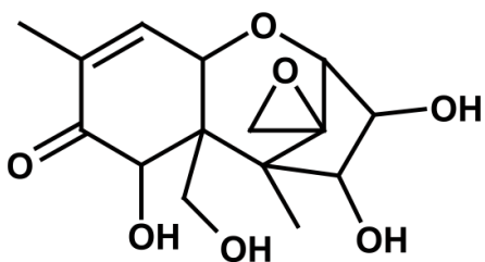
Nivalenol (NIV)
